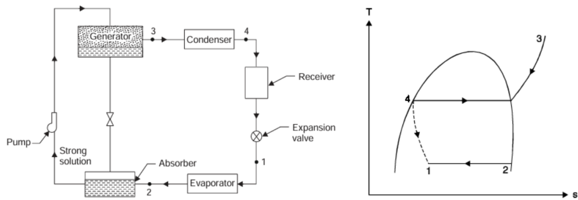
Figura 1.10: Sistema simple de absorción de vapor.
