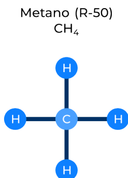
Figura 1.3: Molécula de metano.
